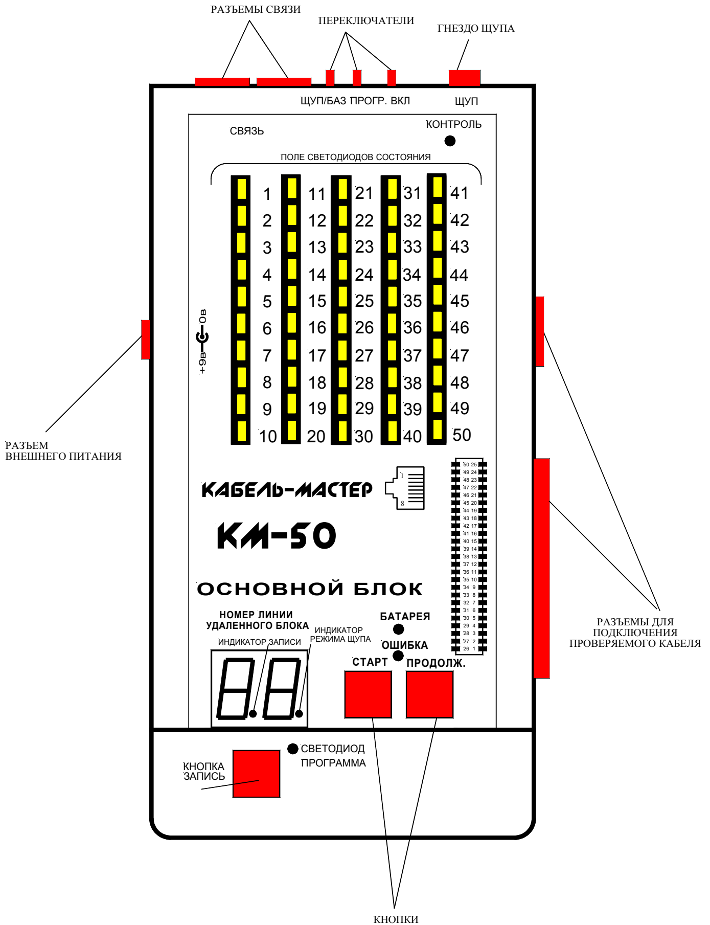
Рис 1. Расположение элементов основного блока.
